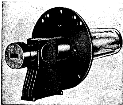
FIG. 19-60.—3J31 magnetron.
